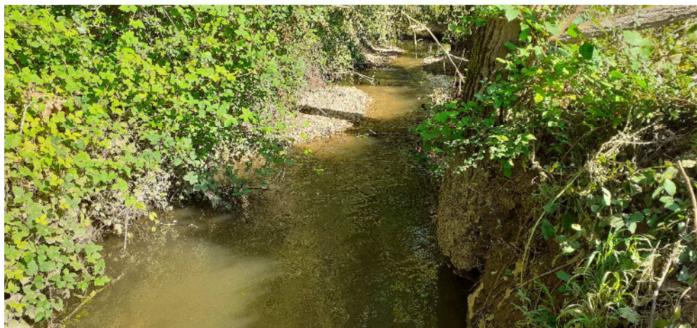
Après les travaux : cours d'eau sinueux et naturel
